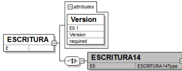
Visión general del esquema XML del tipo de dato ESCRITURA14
