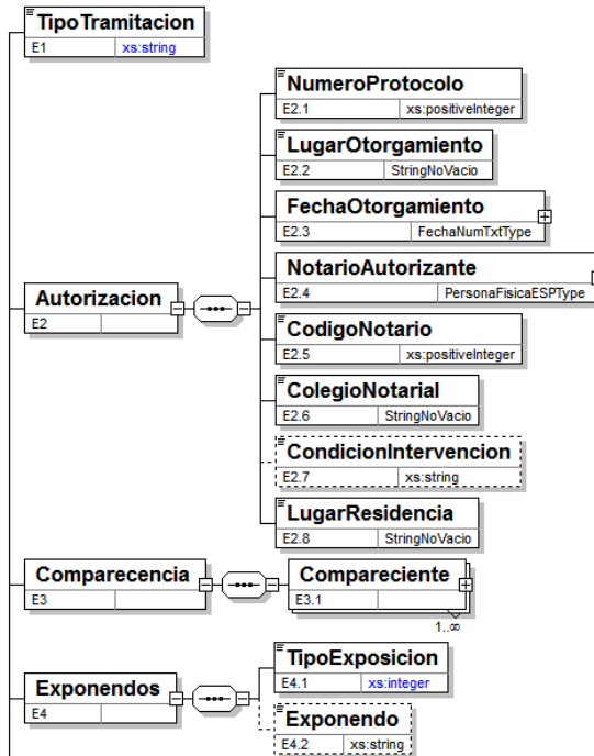
Visión general del esquema XML del tipo de dato ESCRITURA14
